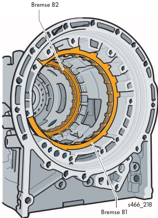
Das Gehäuse des Getriebes mit den eingelegten Lamellen der Bremsen B1 und B2
